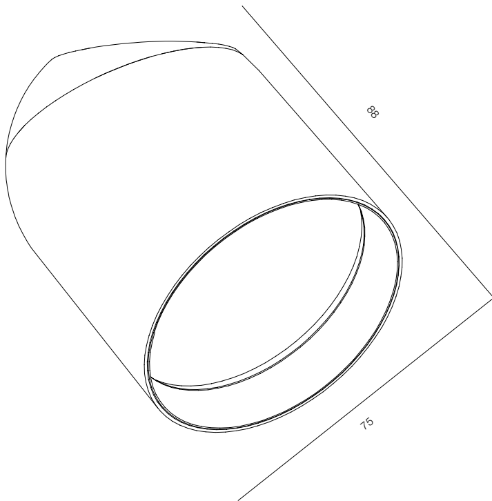
OREO CT COPPA 10W
