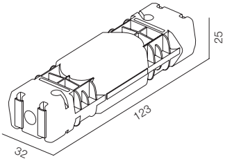
CON 3 PIN IP68 (STB)
