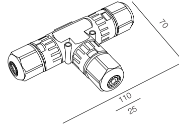
CON T3 PIN IP68
