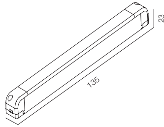
DIM TRIAC 220V LNTC 7W
