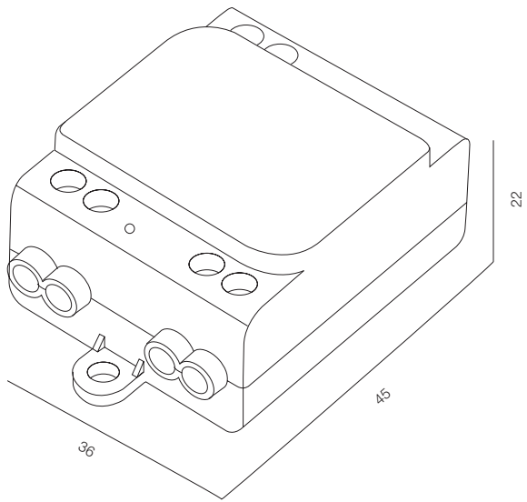
CASAMBI CBU-ASD
