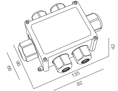
CON PIN IP68 BOX 6
