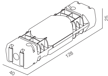
CON 5 PIN IP68 (STB)
