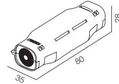
CON 2 PIN IP68 (ETL PX)
